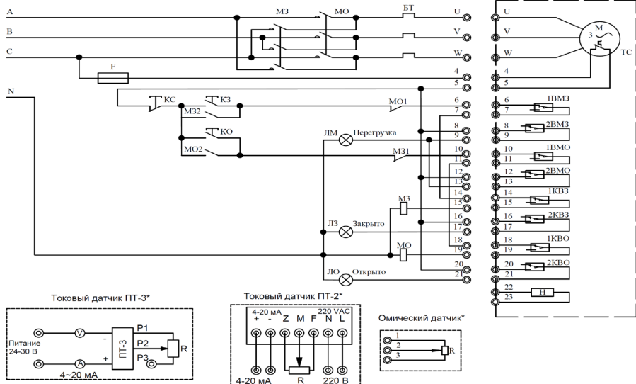
Рис.4 Электрическая схема принципиальная.
