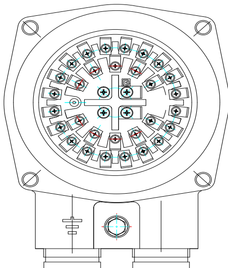
Рис. 6 Взрывозащищенная клеммная коробка
