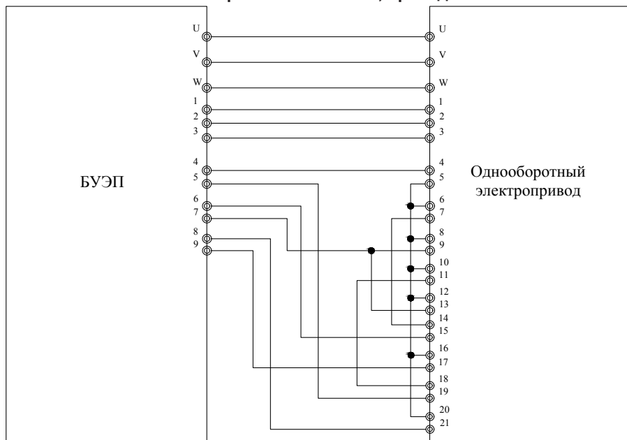
Рис.5 Блок-схема подключения БУЭП к электроприводу
